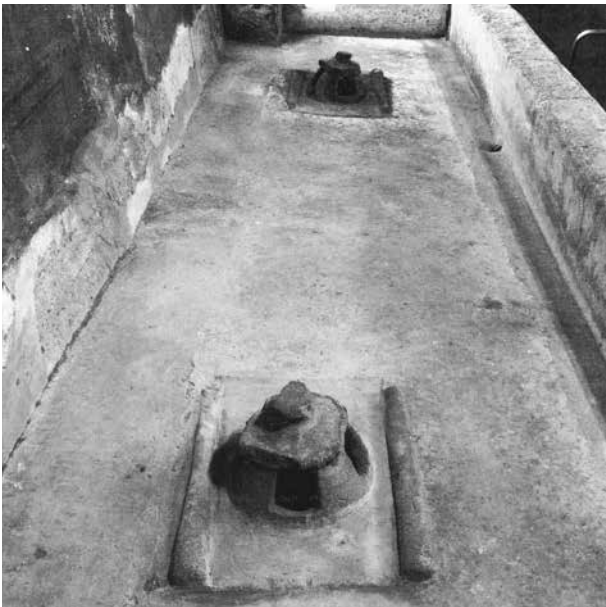
Abb. 35: Pompeji (I), Casa del Centenario (IX 8, 3.6). Zwei Lüftungsziegel auf der Decke der Kryptoportikus.
