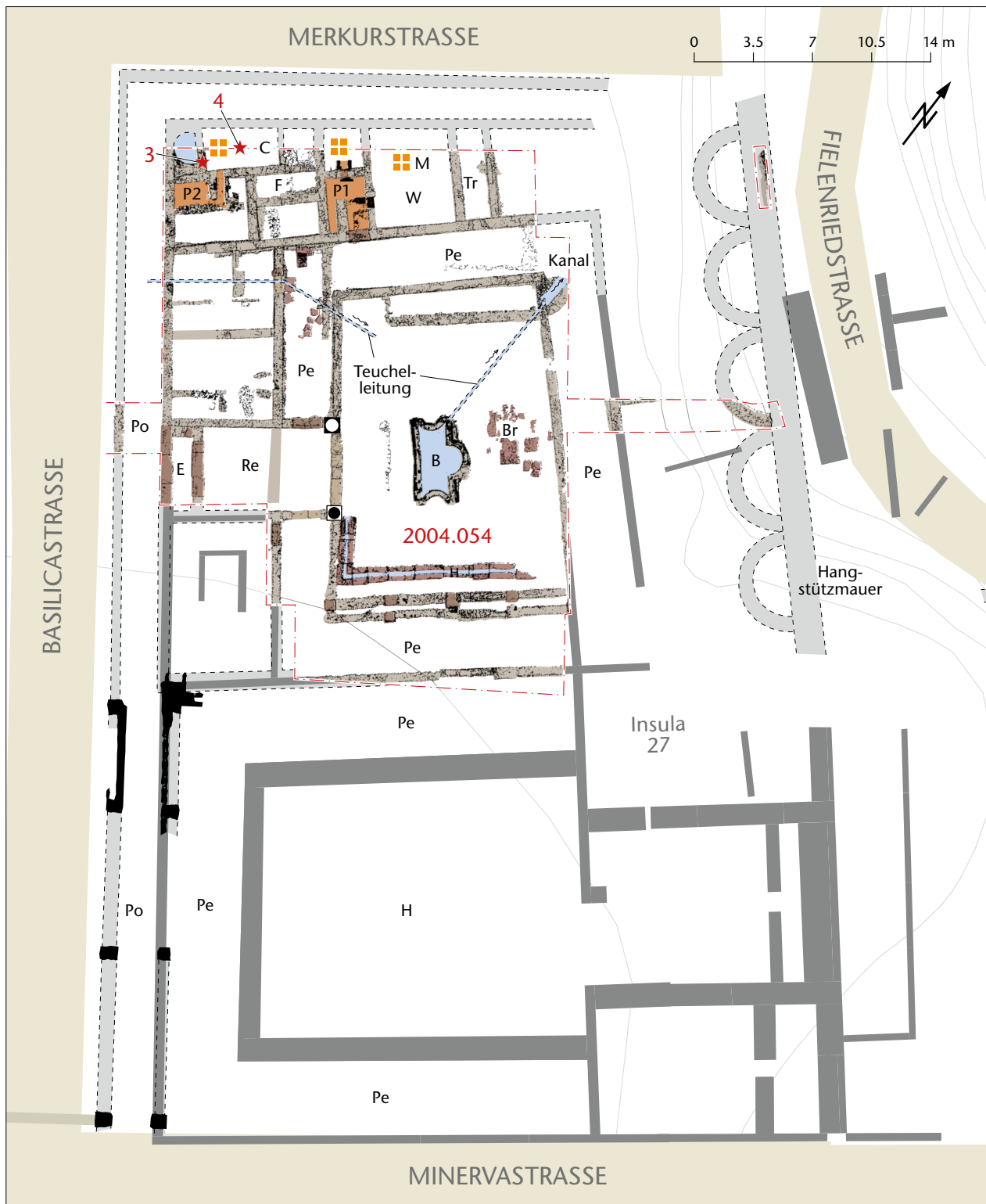
Abb. 28: August BL, Insula 27. Plan des Wohnhauses mit Fundstellen der Ziegelobjekte 3 und 4. M. 1:350.
