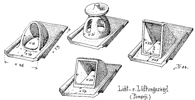
Abb. 34: Lüftungsziegel aus Pompeji (I) mit verschiedenartigen Aufsätzen.
