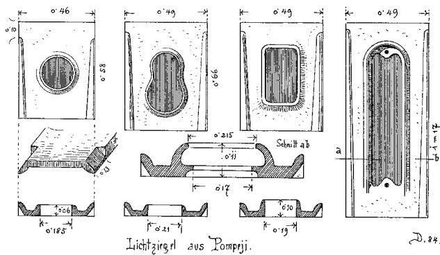
Abb. 33: Lüftungsziegel aus Pompeji (I) mit verschiedenartigen Öffnungen.
